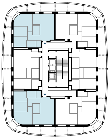
Piso 11 a 12 /13 a 14
